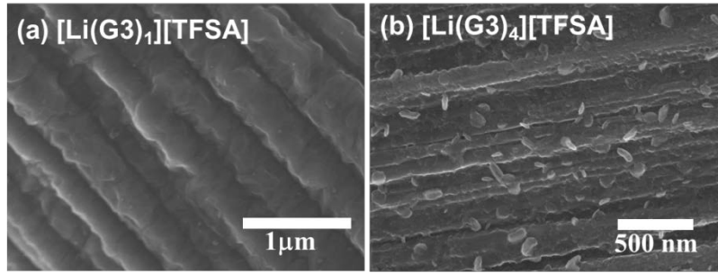
図4 放電反応終了後の正極（カーボンペーパー）上のFE-SEM 観察像（加速電圧: 2 kV）。電解液: (a) 溶媒和イオン液体 [Li(G3) 1 ][TFSA], (b) G3 過剰電解液 [Li(G3) 4 ][TFSA]。トランスファーベッセルを利用。
