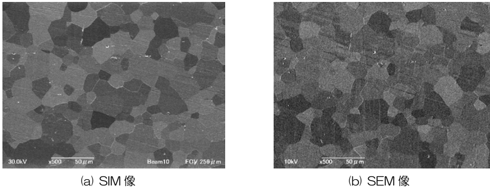
図 6. 同一視野から得た SIM 像および SEM 像
