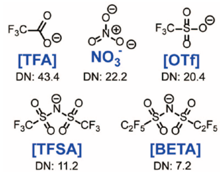
図5 本研究で用いたリチウム塩のアニオン構造とそのドナー数。
