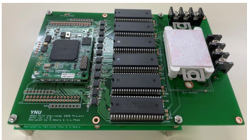
図 2: デジタルオートチューニングユニット (Digital Auto-Tuning Unit: DATU) の試作機
