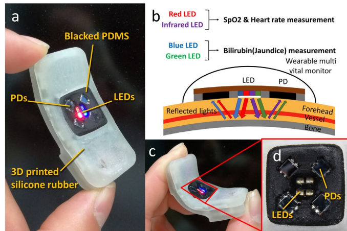
図2 ウェアラブルマルチバイタルセンサの写真： a. 約3センチのセンサ、b. 2つのLEDからの反射光を4つのフォトダイオードで計測、c. デバイス上の小型ICとBluetoothモジュール、d. センサ部分の拡大図
