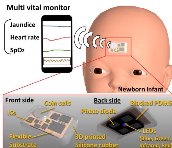
図1 ウェアラブル型マルチバイタルセンサ
