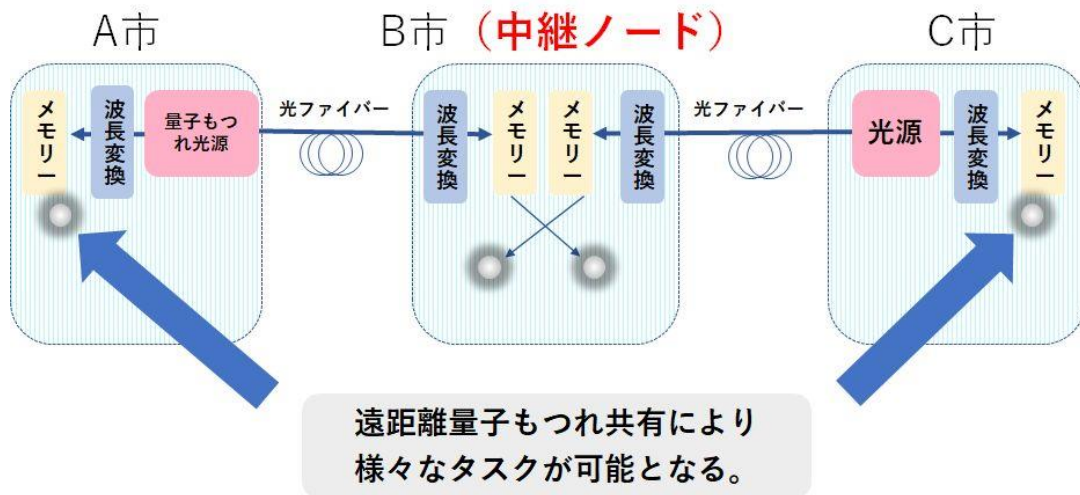
図2：長距離量子通信用量子中継器の概念図。最終的に通信を行いたい2ユーザー間に中継器ノードがあり、ノード間やユーザーを結ぶために2光子源が必要となる。2光子源が中継器ノード搭載メモリと効率よく結ばれるには、狭スペクトル・高輝度の量子もつれ光源および波長変換といった要素が必要となる。
